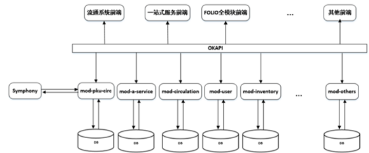
双流通平台架构图
